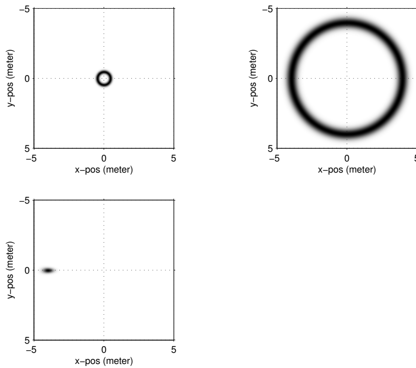
Figur 3.16: Sandsynlighedsfordelingen p(o | x) jf. formel 3.68 for ét landmærke placeret i l = (0, 0) . p_x og p_y varieres i intervallet [-5; 5] . Mørkt svarer til stor sandsynlighed og lyst svarer til lille sandsynlighed.
