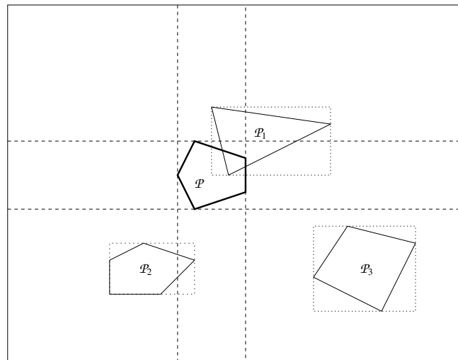
Figur 2.16: Illustration af overlap mellem en polygon P og en mængde af polygoner P_i . Figuren illustrerer tre delfaldende, nemlig P overlapper P_1 , P overlapper ikke P_2 , men de akseparallelle omgivne rektangler for P og P_2 overlapper. P og P_3 overlapper på ingen måde hinanden.
