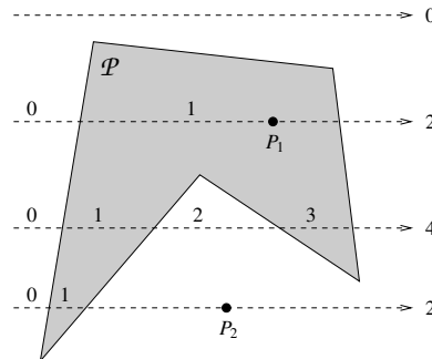
Figur 2.15: Konstatning om et punkt ligger inde i en polygon. Når en stiblet linje følges, tælles antallet t af gange en kant fra polygonen passerer. Gælder t \equiv 1 \pmod{2} , så ligger punktet inde i polygonen.
