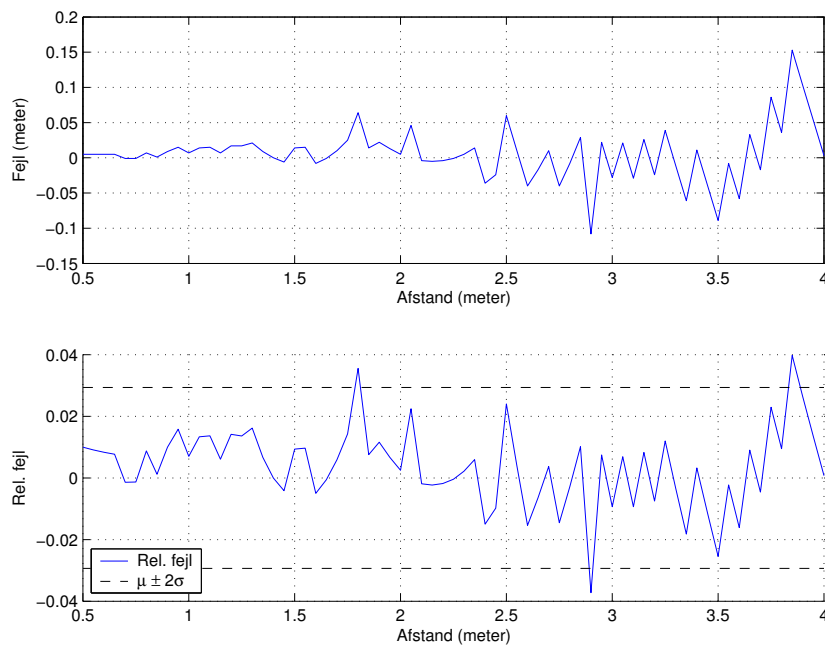
Figur 3.11: Øverst: Fejl i den beregnede afstand som funktion af den reelle afstand til et landmærke. Med fejl menes differencen d - \hat{d} mellem den med kameraet beregnede og den målte afstand.
