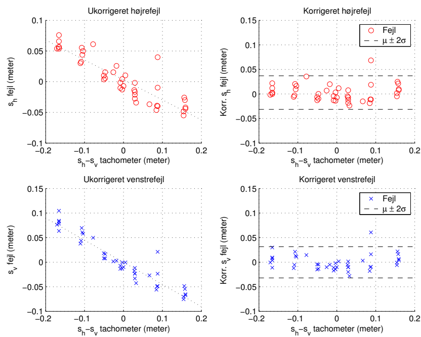
Figur 3.5: De to venstrestående grafer: Fejlen s_h - \hat{s}_h hhv. s_v - \hat{s}_v i den kørtte strækning som funktion af differencen s_h - s_v .
