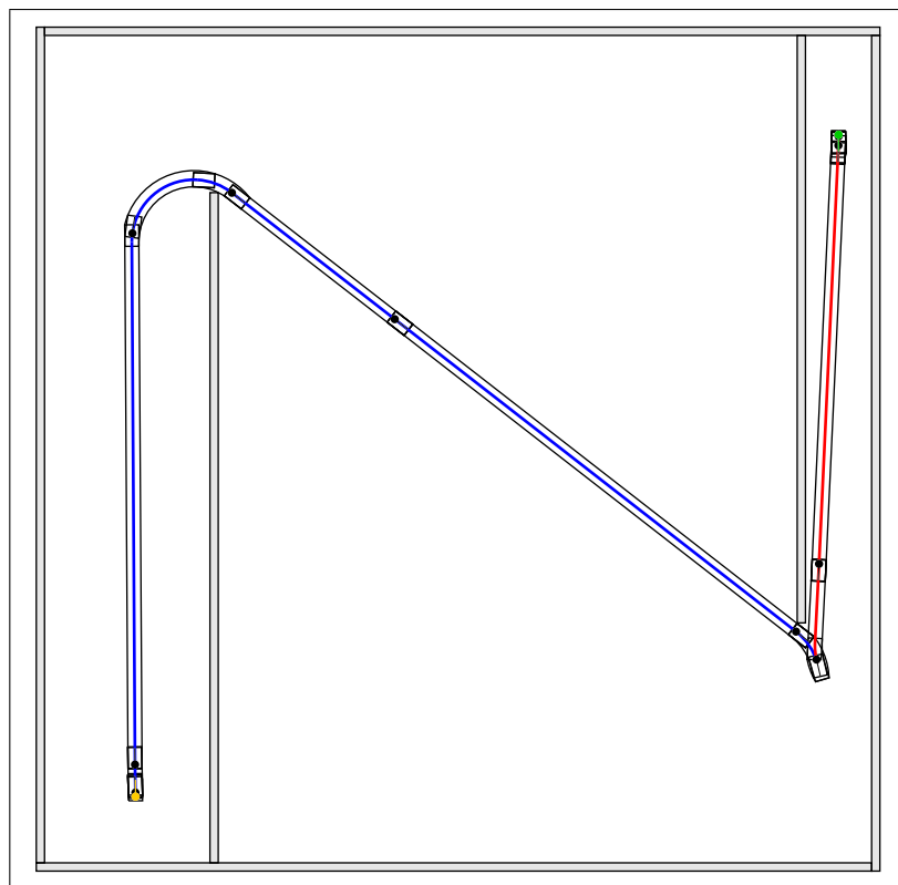
Figur 2.27: Kort med to korridorer. Specielt den højre korridor er udfordrende for ruteplanlægningen, da den er meget smal. Den er lige netop bred nok til at robotten kan vende inde i korridoren.
