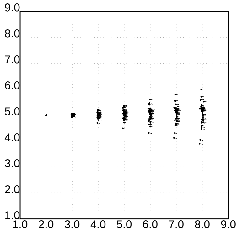
Figur 3.14: Eksempel på anvendelse af bevægelsesmodellen ved kørsel ligeud. Startpositionen initialiseres til x_0 = (2, 5, 0) . Formel 3.57 og formel 3.55 bruges til at opdatere positionen, som er vist for hver meter, indtil 6 meter er kørt. Dette er gentaget 50 gange. Spredningen er givet ved \Sigma_1 .
