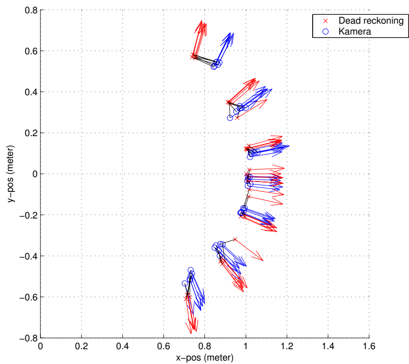
Figur 3.2: Den ud fra kameraets målinger beregnede position, samt positionen beregnet ud fra robottens tachometermålinger. Korresponderende positioner er forbundet med sorte linjer.
